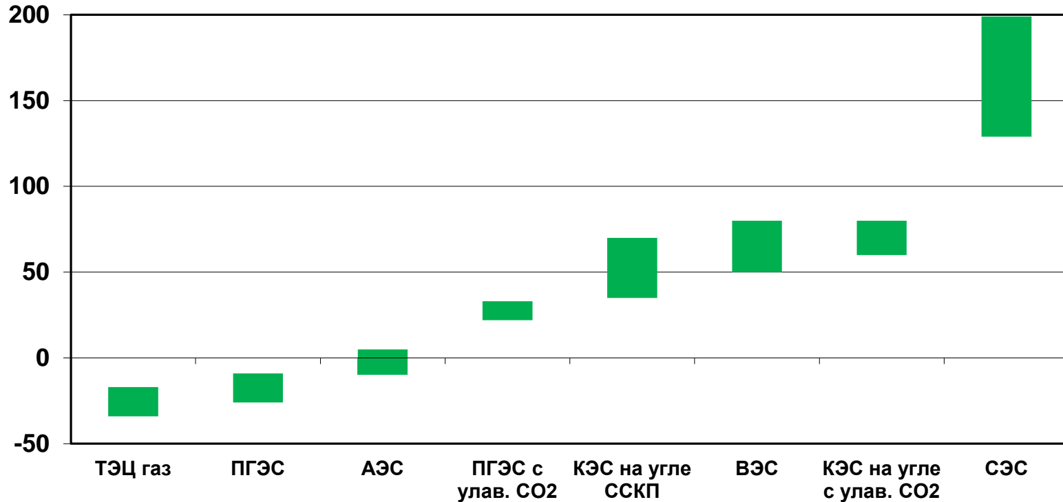
Стоимость избегаемых выбросов, долл. 2013/т CO 2
