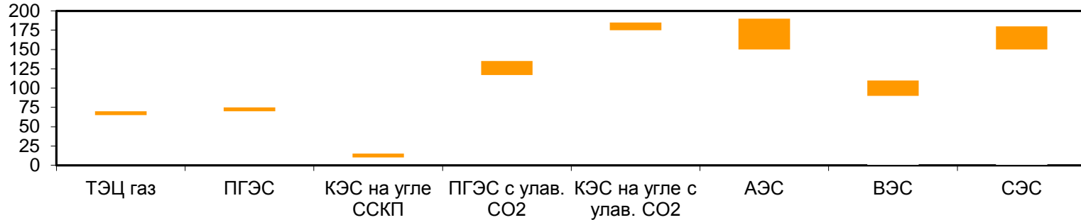
Удельные выбросы CO2 и снижение относительно КЭС 24 МПа на угле, т/МВт.ч
