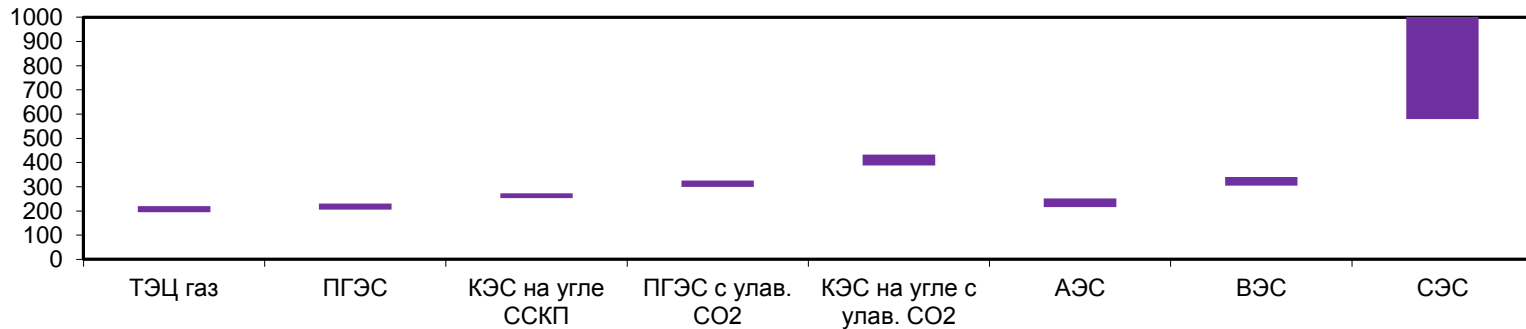
Удельные дисконтированные затраты на производство электроэнергии, коп.2013/кВт.ч
