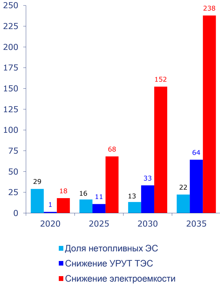
Факторы сдерживания эмиссии ПГ, млн т CO 2 -экв
